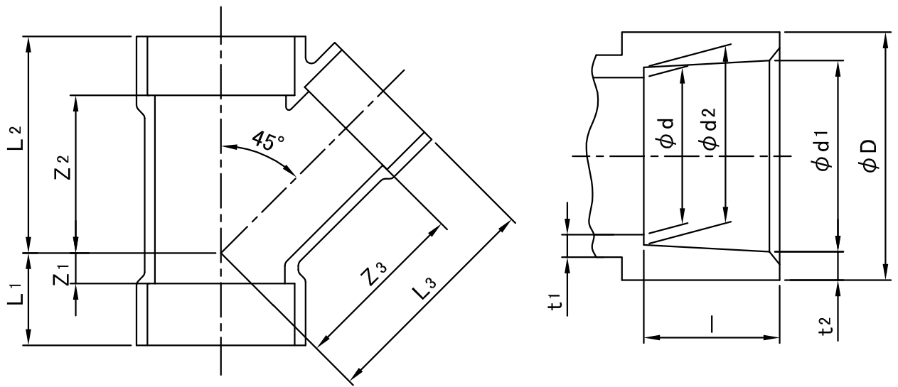
接合部寸法
