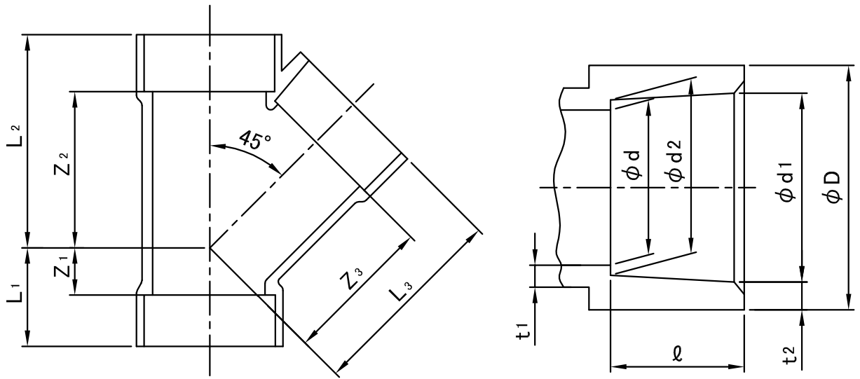
接合部寸法
