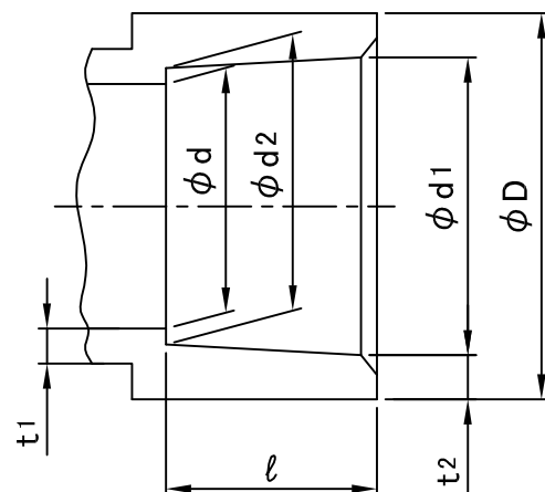
接合部寸法
