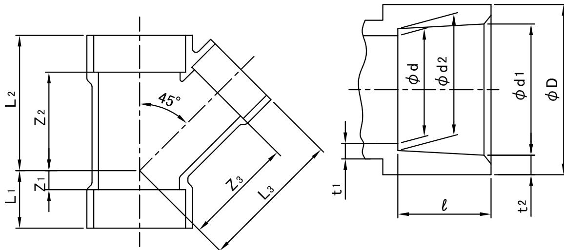
接合部寸法
