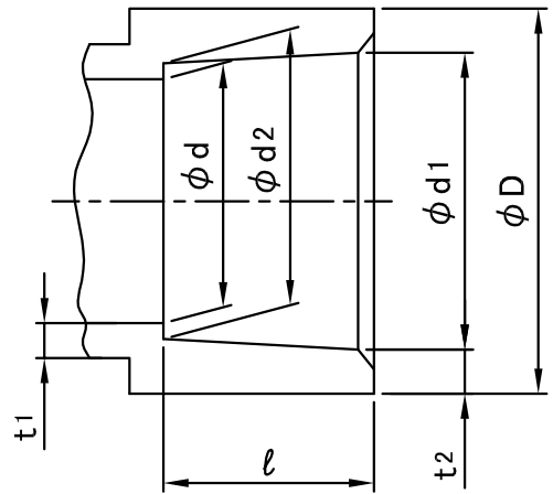
接合部寸法
