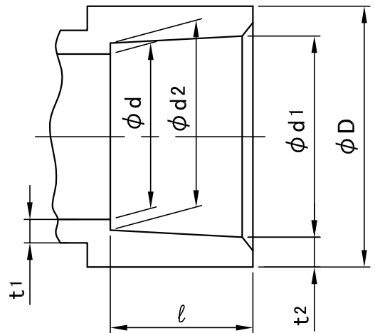
接合部寸法
