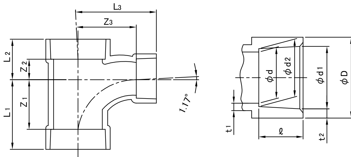
接合部寸法
