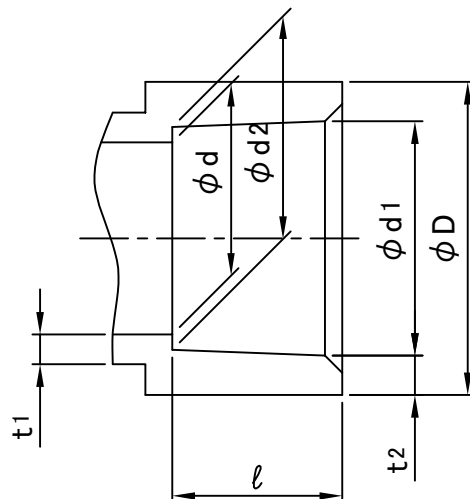
接合部寸法
