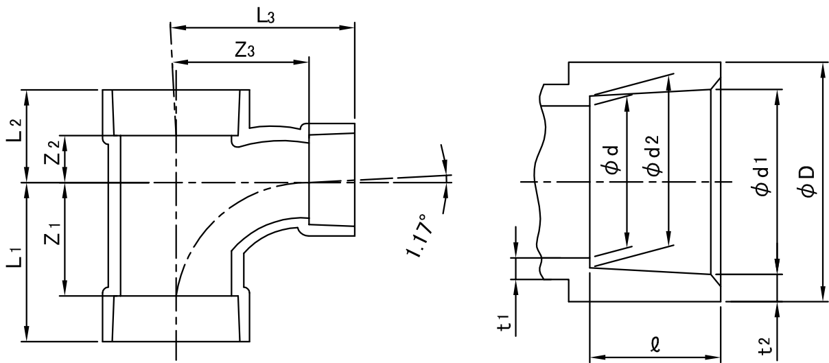
接合部寸法
