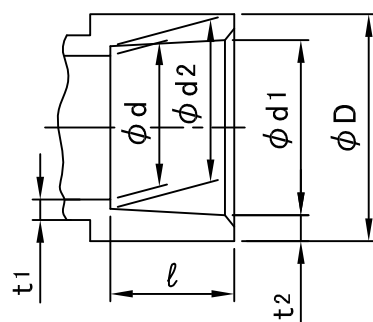
接合部寸法
