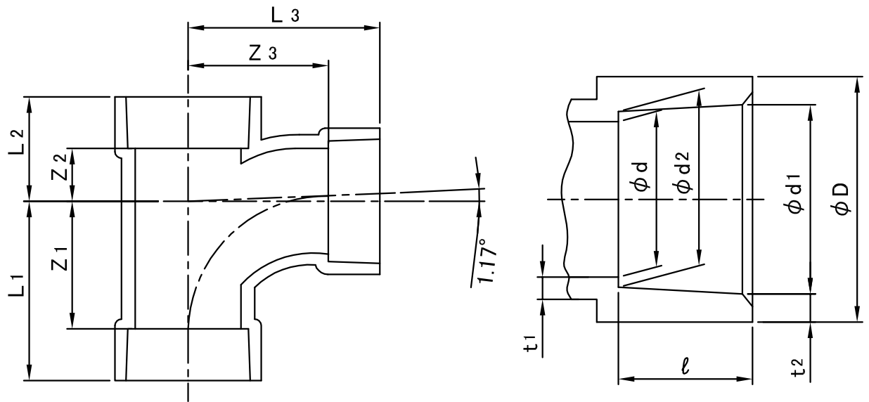
接合部寸法
