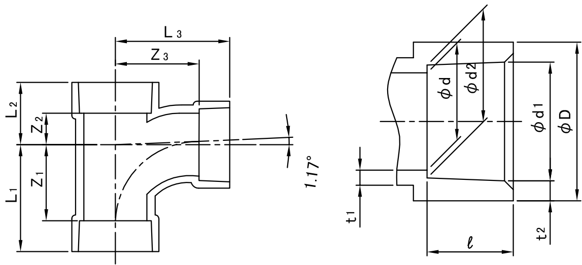
接合部寸法
