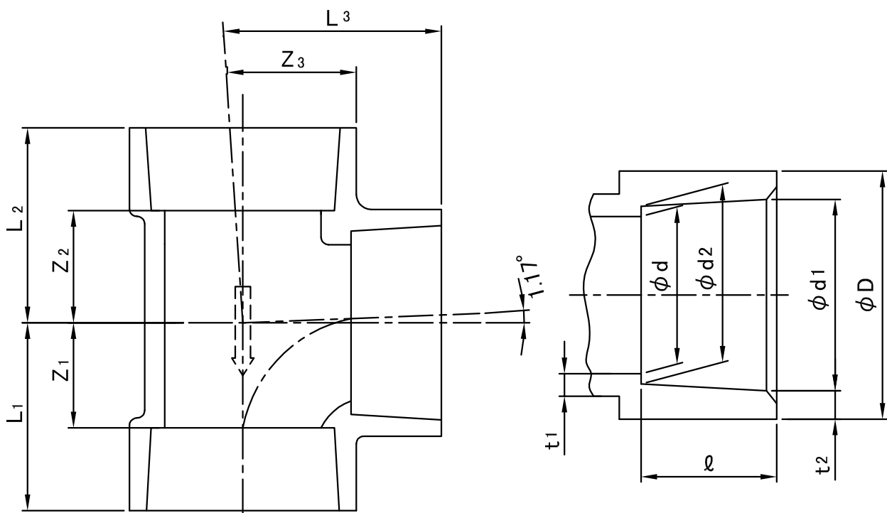
接合部寸法
