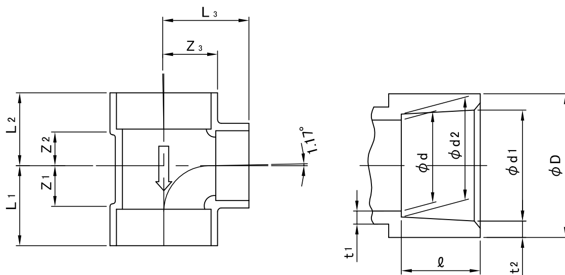
接合部寸法
