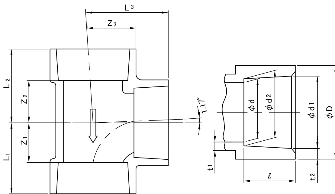
接合部寸法
