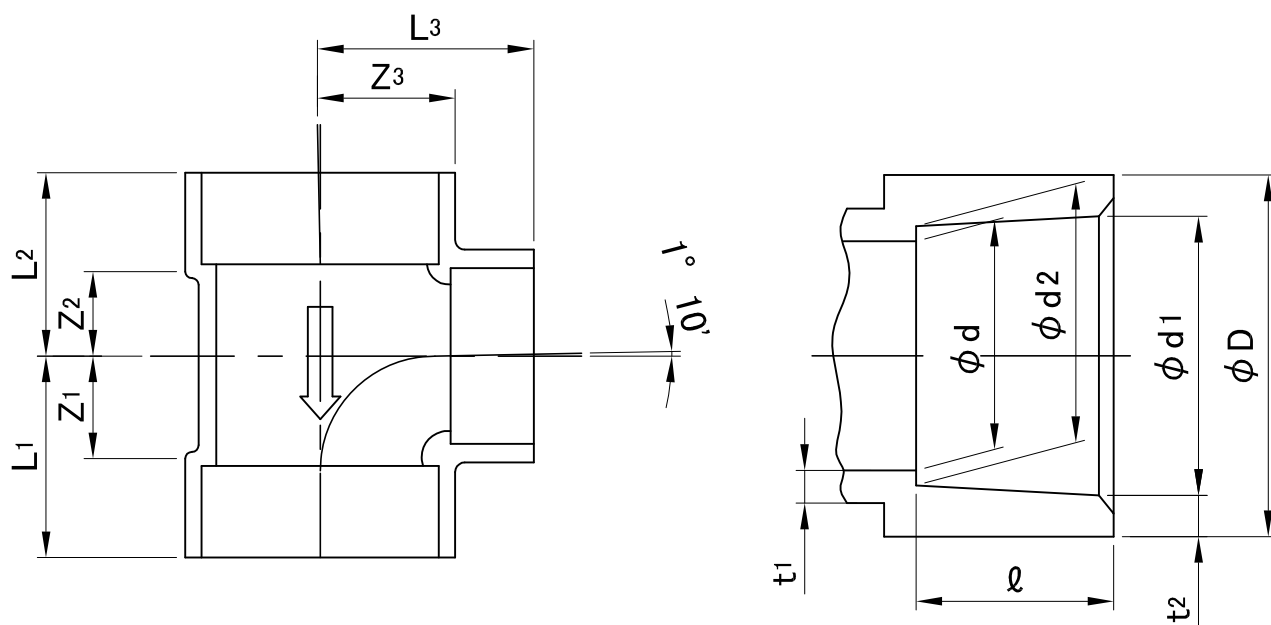
接合部寸法
