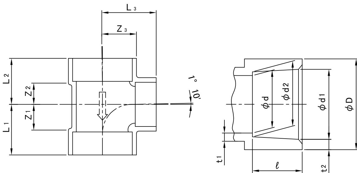
接合部寸法
