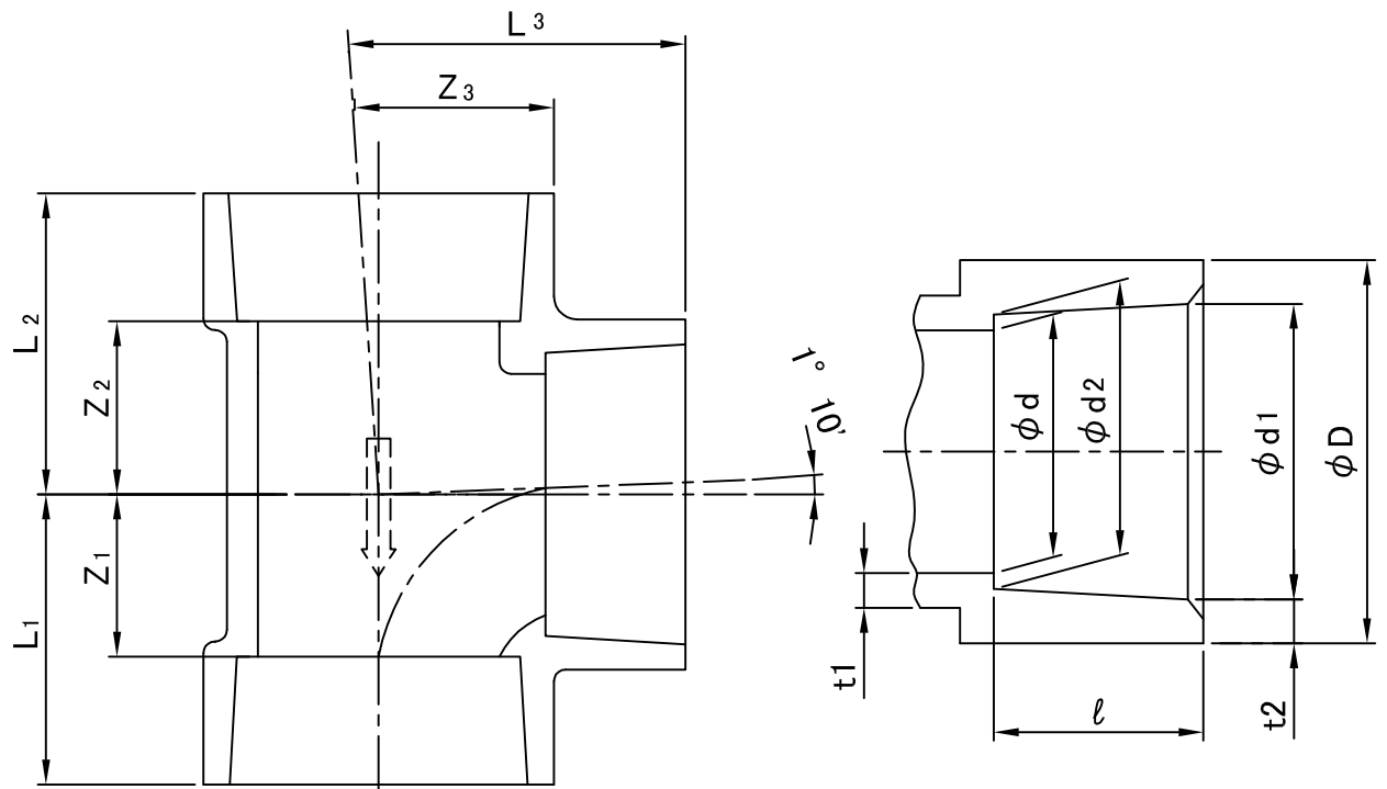
接合部寸法
