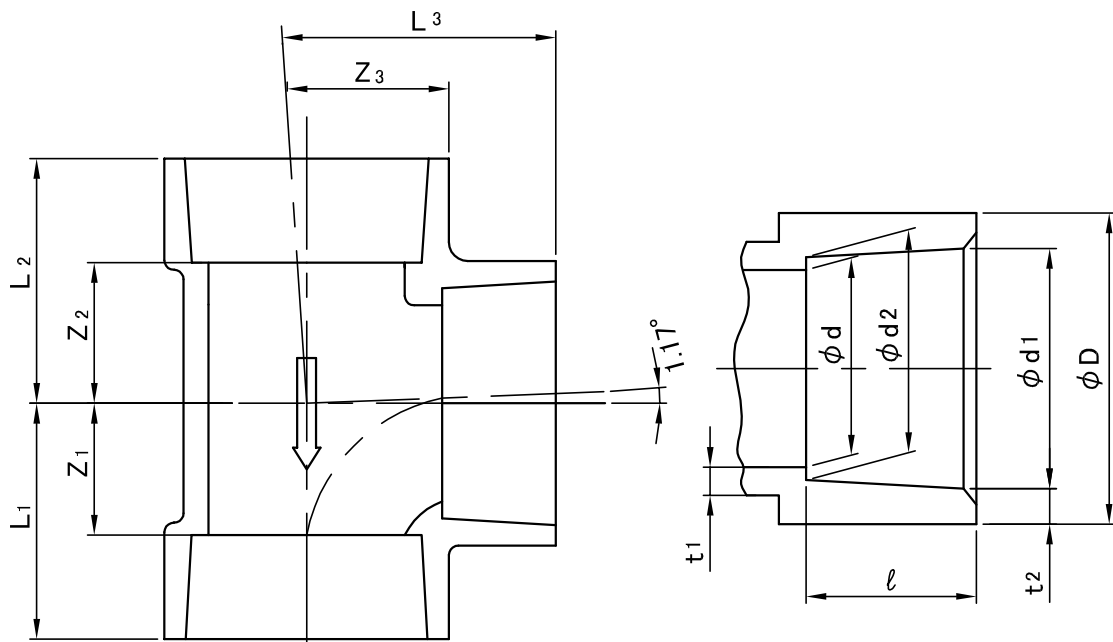
接合部寸法
