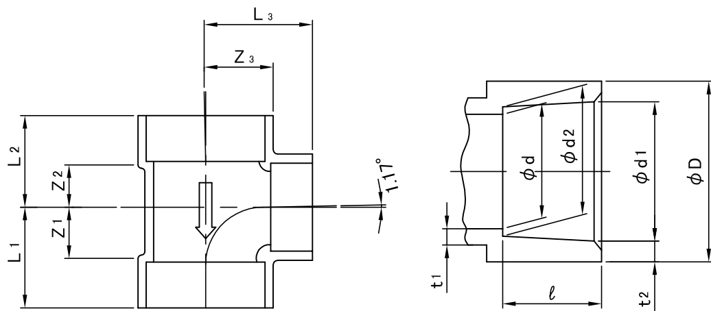
接合部寸法
