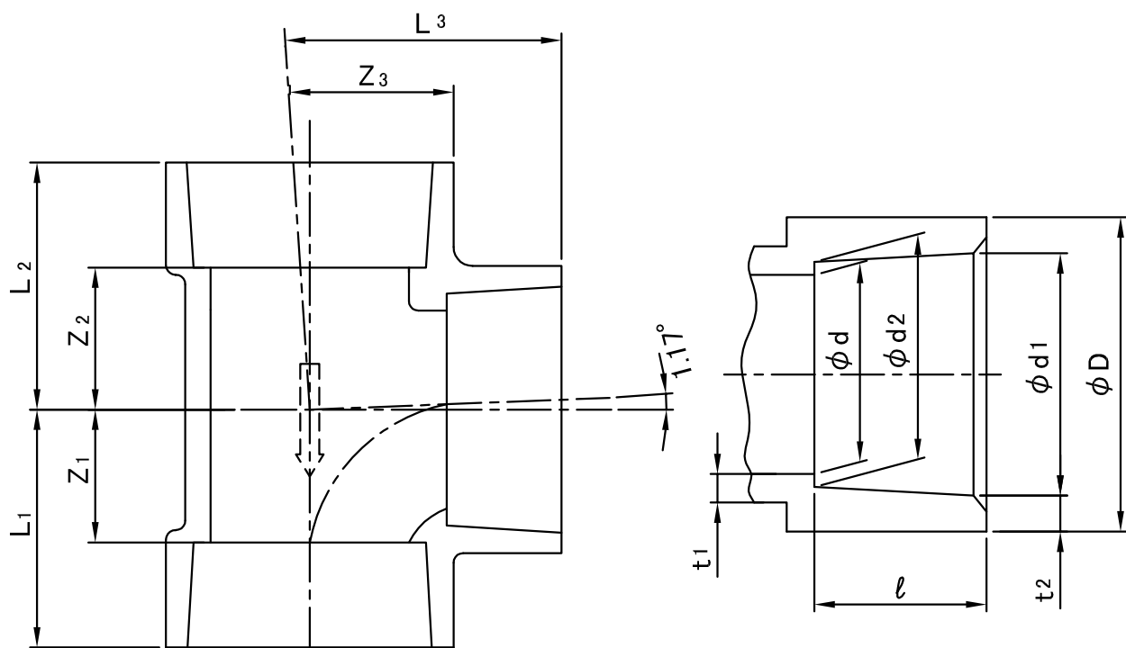
接合部寸法
