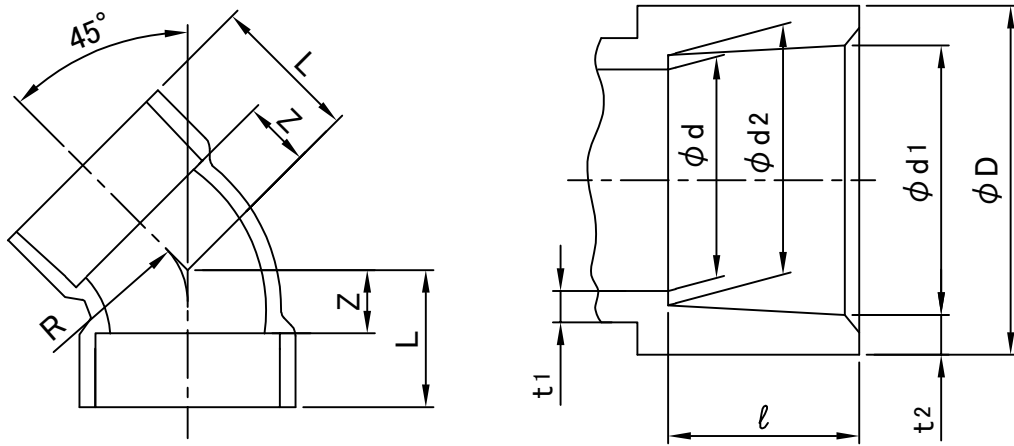
接合部寸法
