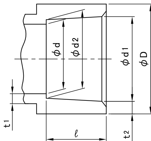
接合部寸法
