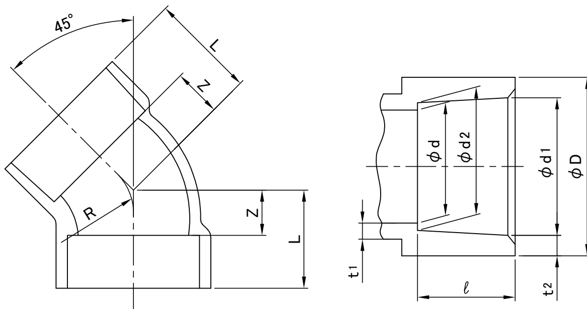
接合部寸法
