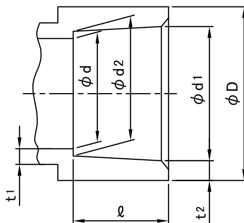
接合部寸法
