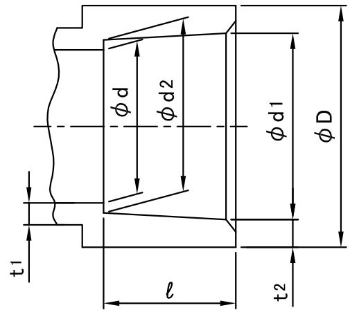
接合部寸法
