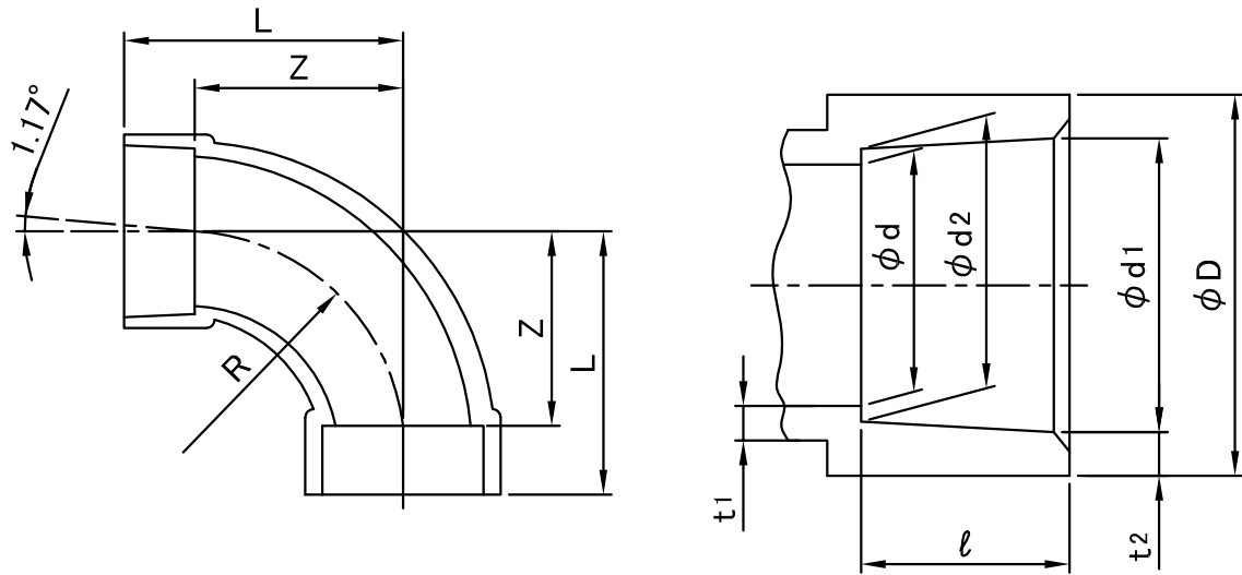
接合部寸法
