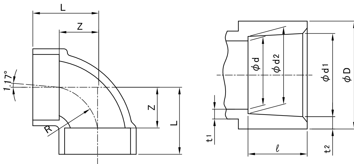
接合部寸法
