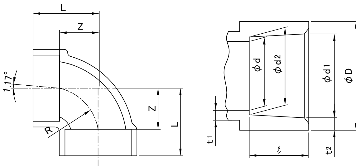
接合部寸法
