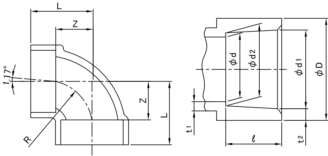
接合部寸法
