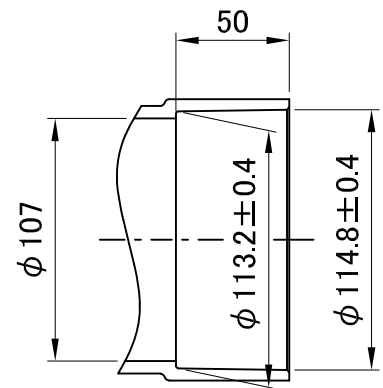
キャップ挿入部受口寸法図
