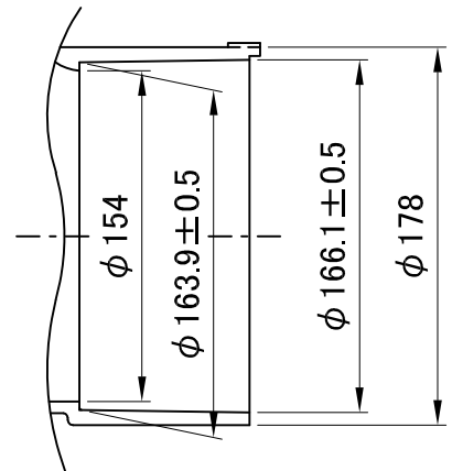
キャップ挿入部受口寸法図
