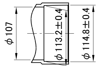
キャップ挿入部受口寸法図
