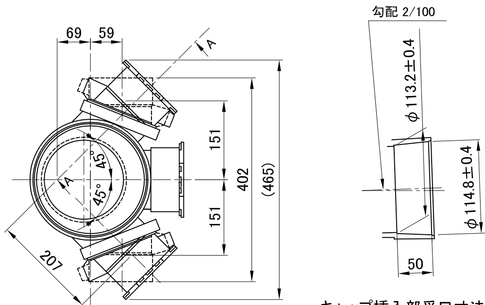
キャップ挿入部受口寸法図
