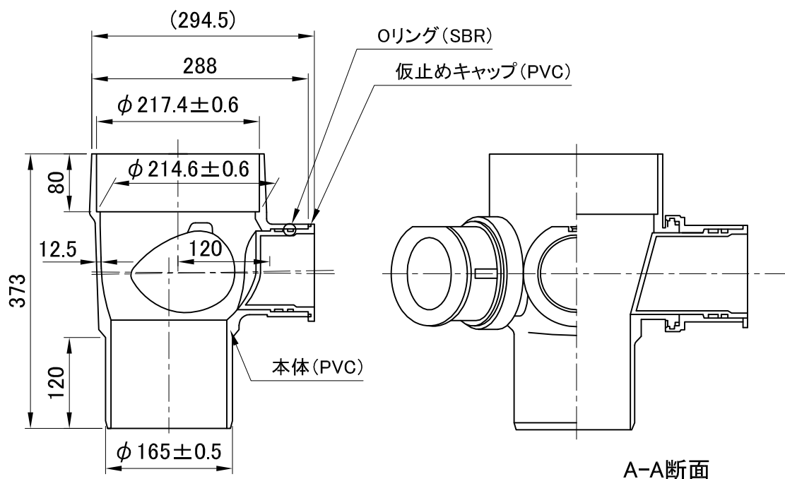
キャップ挿入部受口寸法図
