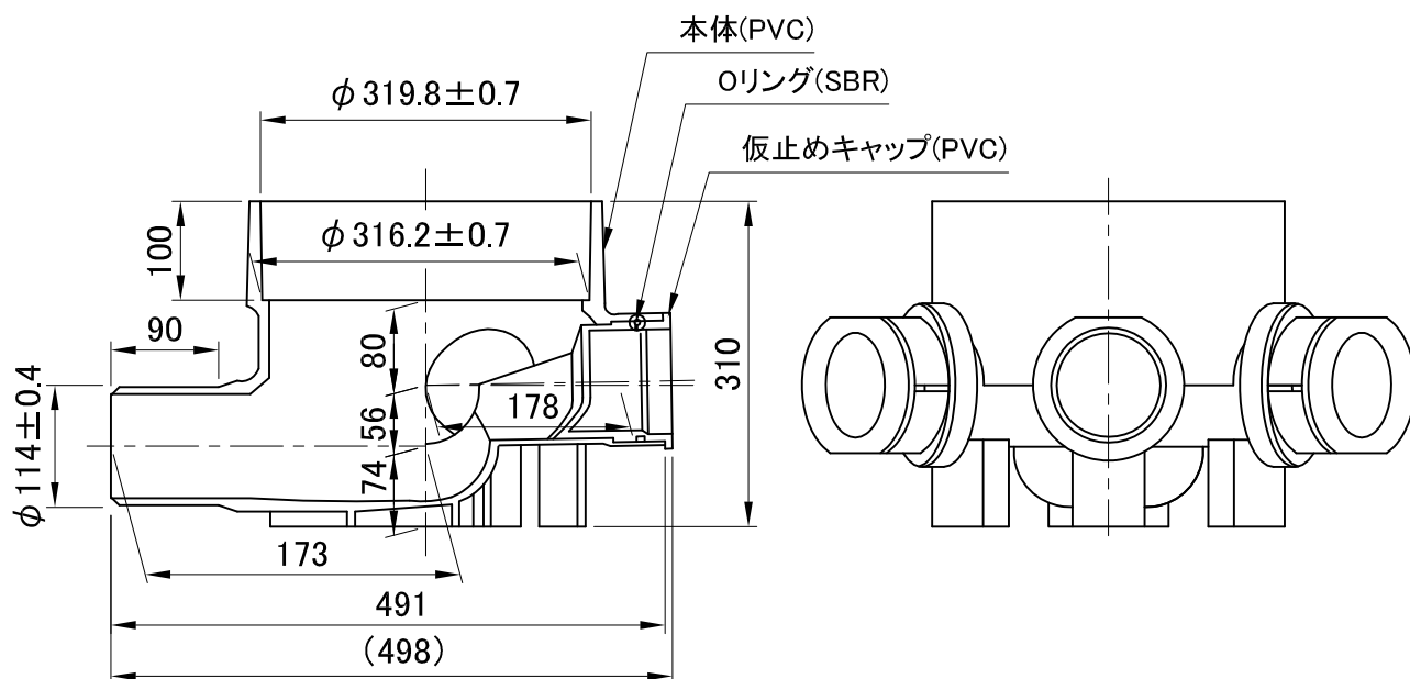
キャップ挿入部受口寸法図
