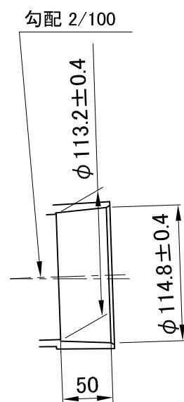
キャップ挿入部受口寸法図
