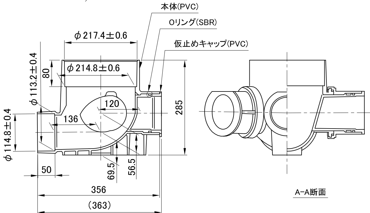
キャップ挿入部寸法
