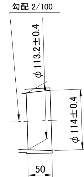
キャップ挿入部寸法
