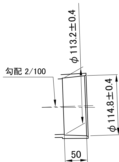
キャップ挿入部受口寸法図
