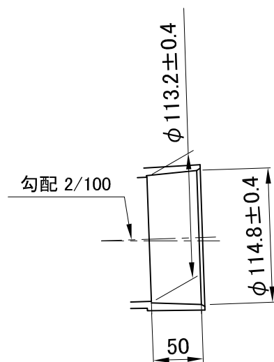
キャップ挿入部寸法
