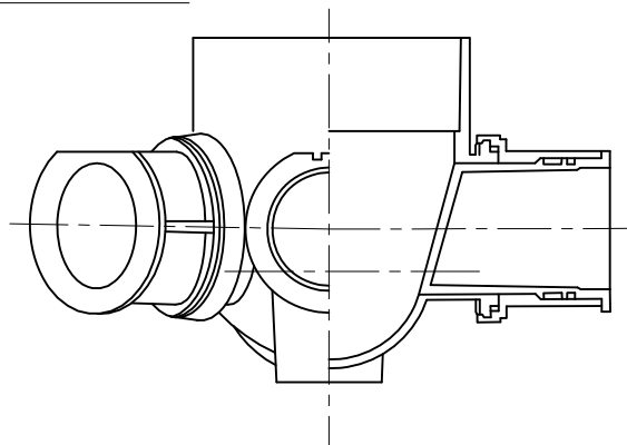
A-A断面
