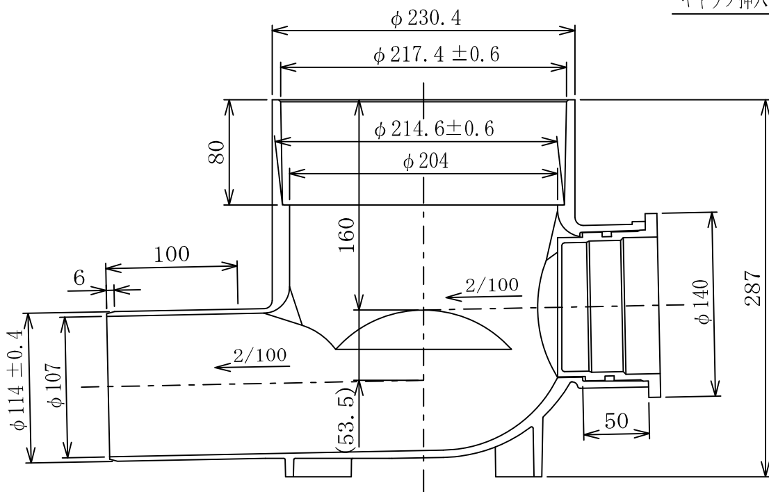
キャップ挿入部受口寸法図
