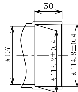
キャップ挿入部受口寸法図
