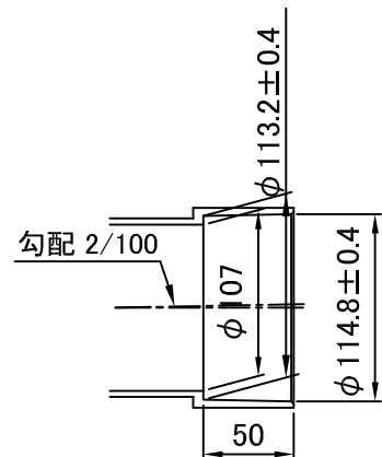
キャップ挿入部受口寸法図
