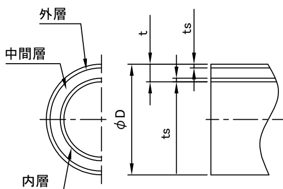
断面(直管部)拡大図
