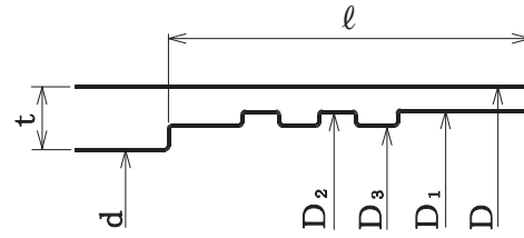
受口部詳細図
